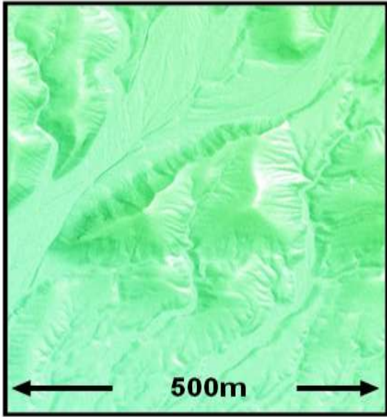
LiDAR DEM
